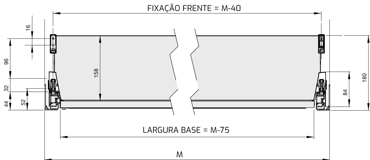
Gaveta H84 com tubo lateral - traseira de gaveta alta.
