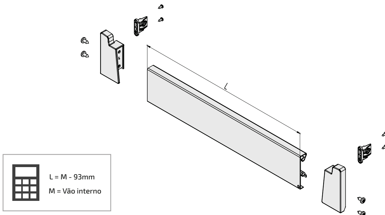
Frente da gaveta interna (montagem)
